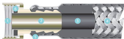
1 Latón niquelado. 2 Latón. 3 Caucho EPDM. 4 Malla estándar acero inox. 5 Acero inox. 6 Caucho EPDM.
